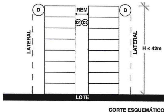
CORTE ESQUEMÁTICO
