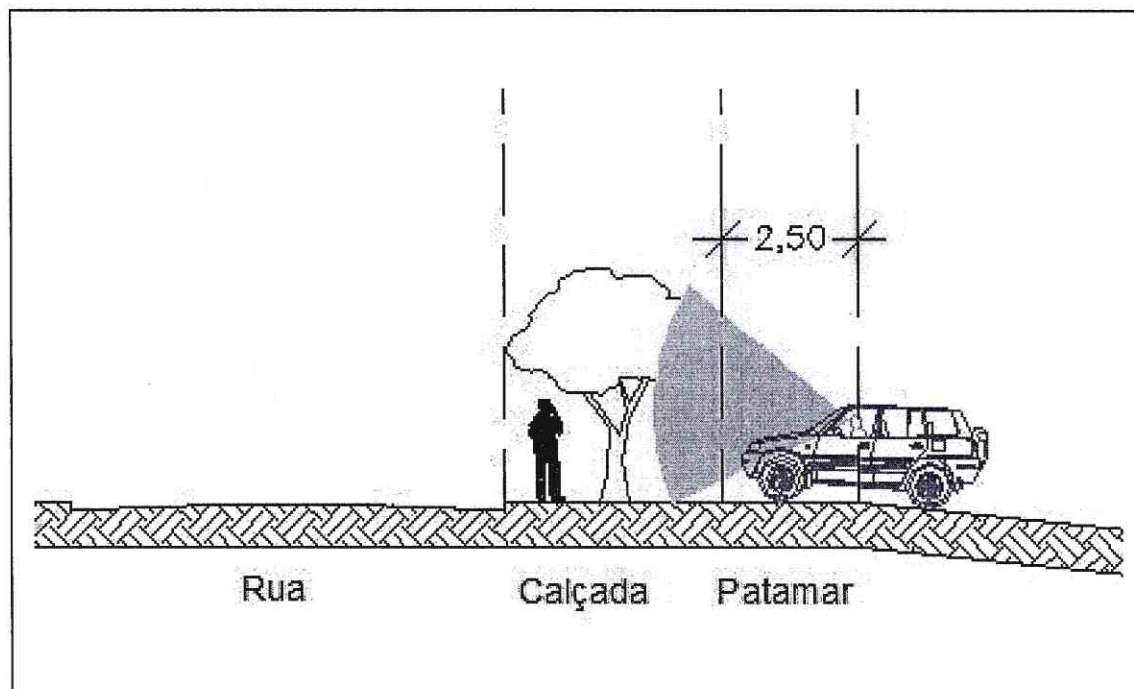
FIGURA 1 - RECUO DAS RAMPAS PARA AUTOMÓVEIS
