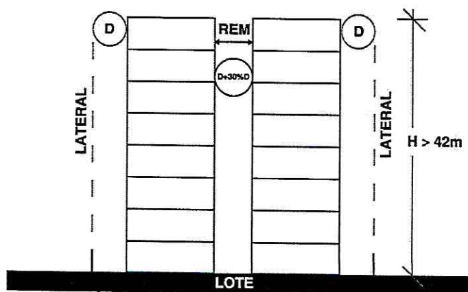
CORTE ESQUEMÁTICO
